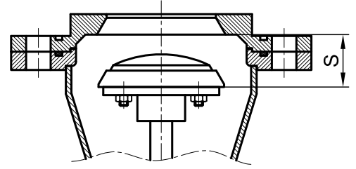
Strok pozisyonu
